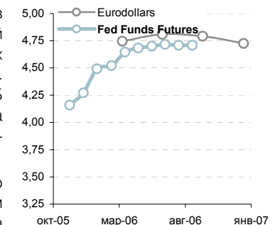
Кривая фьючерсов на процентную ставку
